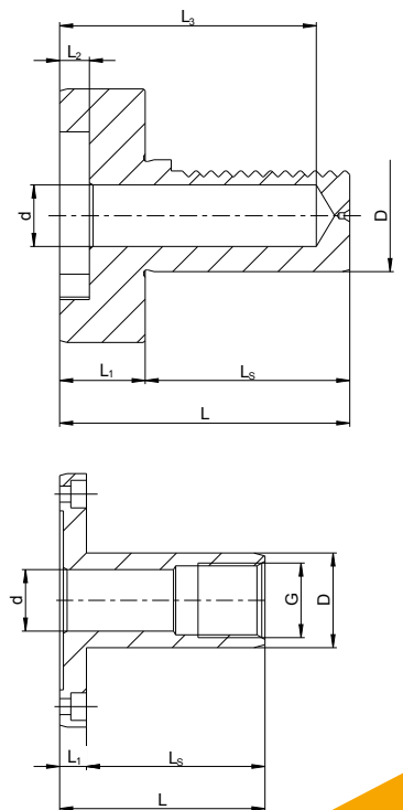
Abbildung: Schaftmaße, siehe Tabelle
